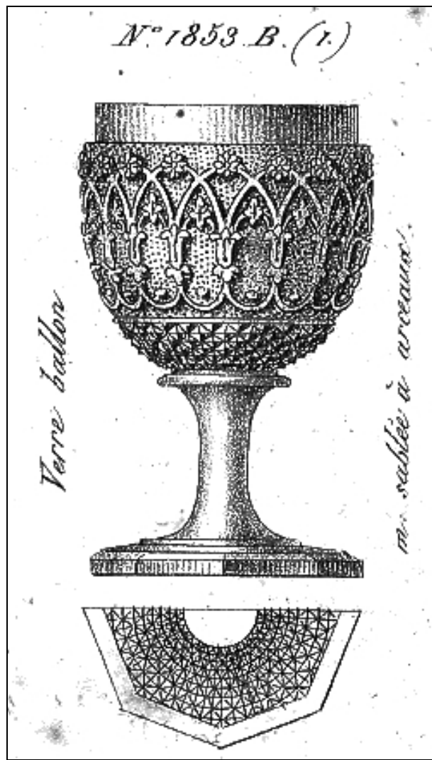
Abb. 2001-05/378 (Ausschnitt) MB Launay, Hautin & Cie., um 1840, 2. me Partie: Planche 52, Service de Table. Moulure sablée et guirlande, No. 1853 B. (1), Verre ballon m. sablée à arceaux, Baccarat 1840 MB Sammlung CMOG
