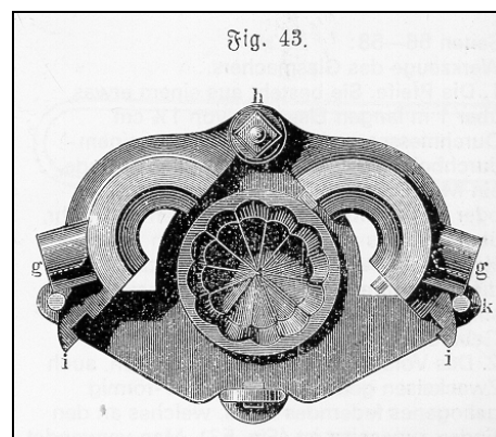
Abb. 1999-5/096 und Abb. 1999-5/102 Fig. 43, Pressform, Draufsicht bei geöffnetem Deckring die Positiv-Form ist dreh-symmetrisch, das Oberteil der Negativ-Form kann mit einer ebenen Nahtfläche durch die Zentral-Achse einmal geteilt werden: der einfachste Fall Ober- und Unterteil können rationell nur durch Abguss von einer Positiv-Form aus Metall gewonnen werden Fig. 44, Pressform, Längsschnitt hier zum Blasen in die Form, entweder mit der Glasmacher-Pfeife, einer Luftpumpe oder mit Pressluft! aus Gerner 1897 ; zit. n. Neuwirth 1973 , S. 70 f.
